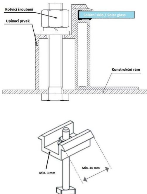
Obrázek č. 4 – Příklad upínání z boční strany a středové upínání pro dva panely vedle sebe
