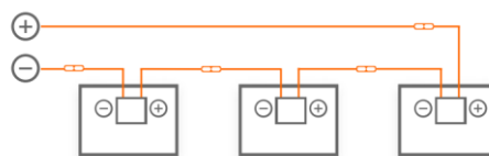
Sériové zapojení
