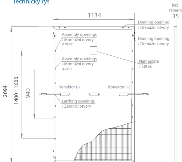
Obrázek č. 2 - Technický výkres panelu řady 380
