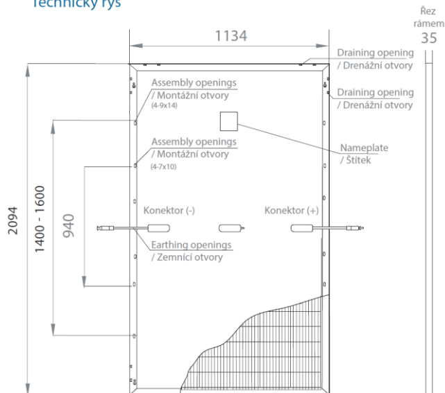
Obrázek č. 2 - Technický výkres panelu řady 500
