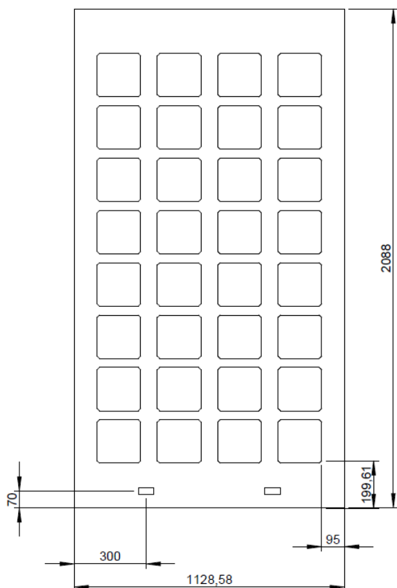
Obrázek č. 2 - Technický výkres panelů řady FT 200 – 450 W
