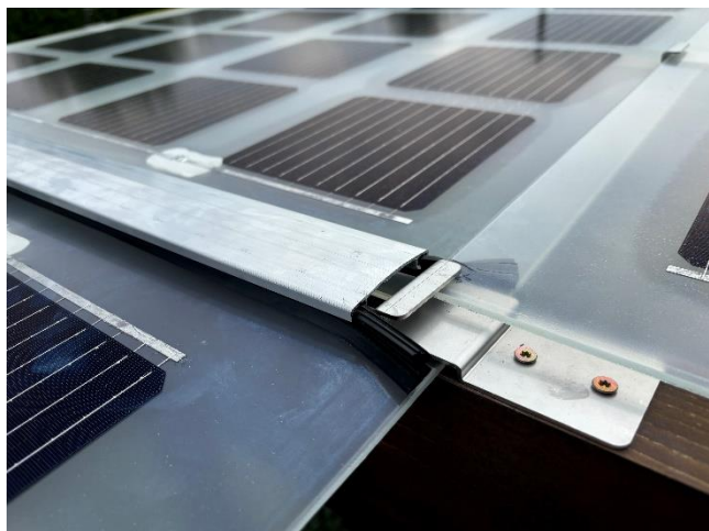
Obrázek 5 – Uložení panelu z boku a navázání horní řady
