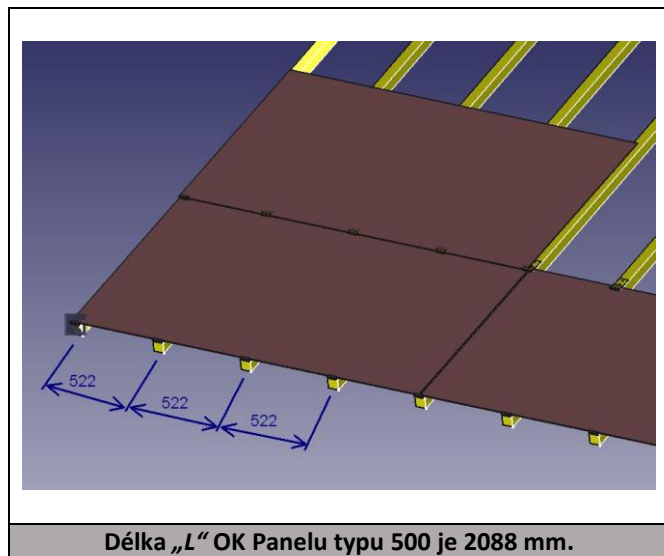
Obr. Rozložení nosníků pro horizontální podepření
